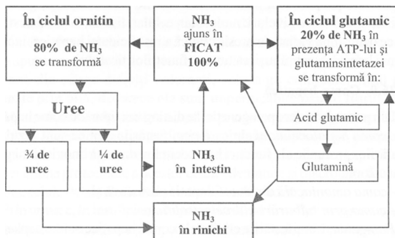
Circuitul schematic al \text{NH}_3 , în organism.
